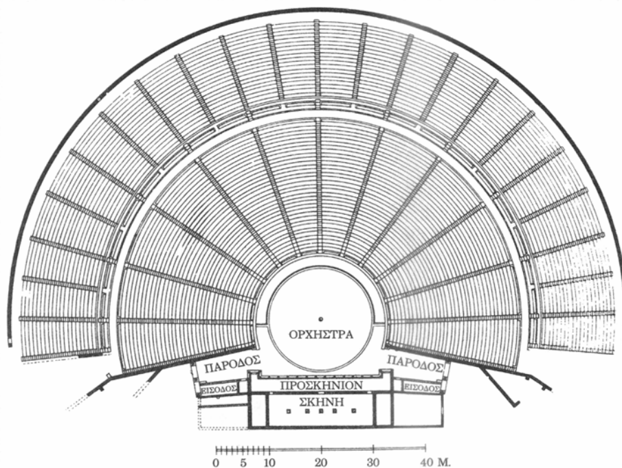
Το θέατρο της Επιδαύρου κάτωψη.
