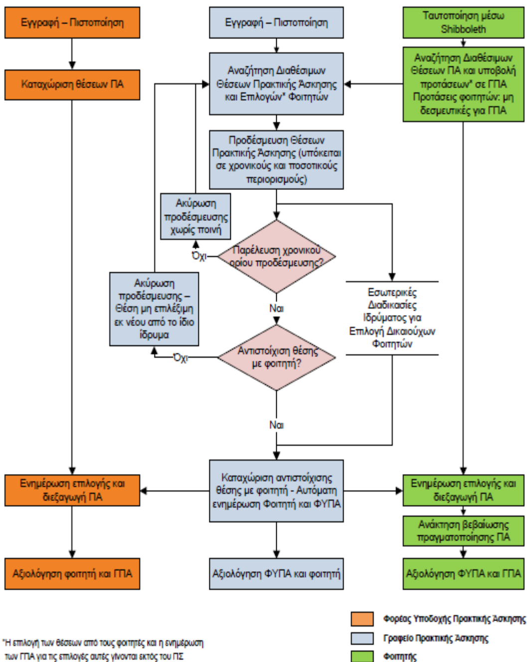
Εικόνα 2.1: Διάγραμμα ροής λειτουργιών
