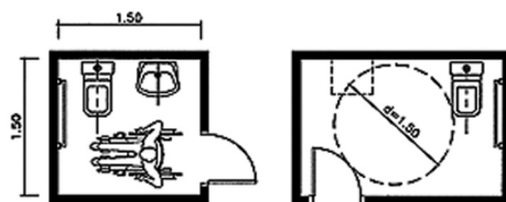
Χώρος πλήρους περιστροφής
