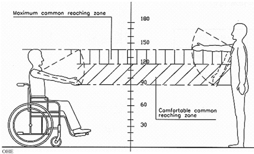
Περιοχές με δυνατότητα προσέγγισης από άτομο σε αναπηρικό αμαξίδιο και όρθιο άτομο
