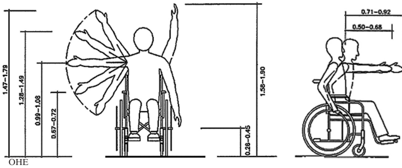
Περιοχή προσεγγίσιμη από άτομο σε αναπηρικό αμαξίδιο
