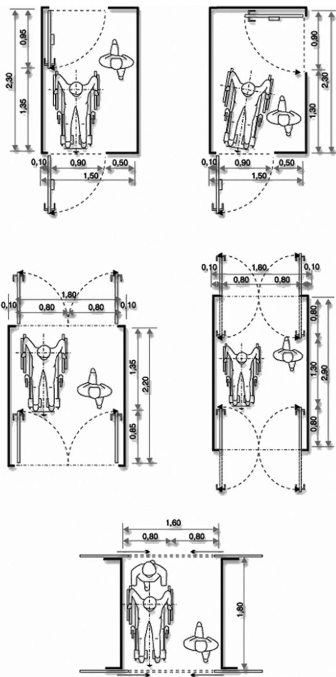
Σχεδιασμός προσβάσιμων ανεμοφρακτών εισόδου
