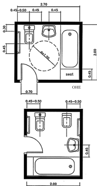
Χωροθέτηση ειδών υγιεινής σε περίπτωση ύπαρξης μπανιέρας
